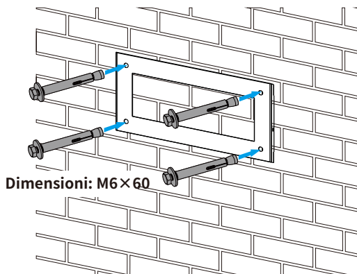
Installazione della staffa di montaggio dell'inverter
