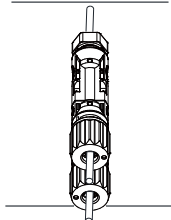
Fig. 3.6 Collegamento ingresso CC
