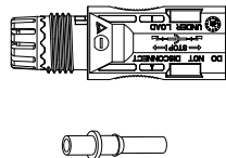
Fig. 3.2 Connettore CC- femmina
