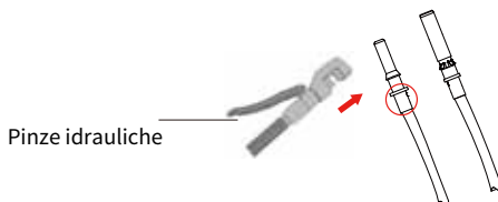
Fig. 5.4 Crimpare il perno di contatto sul filo
