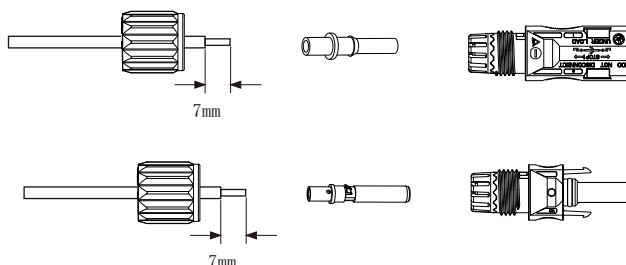
Fig. 5.3 Smontare il dado del cappuccio del connettore
