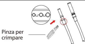
Fig. 5.4 Crimpare il pin di contatto sul filo
