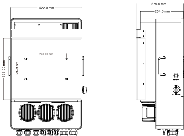
Dimensioni dell'inverter
