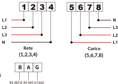
Figura 7.1 Contatore Eastron
