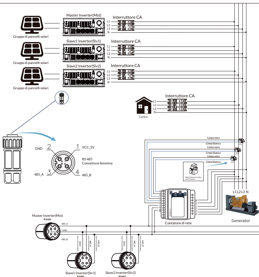
Figura 7.27 Schema di collegamento (elettricità trifase)
