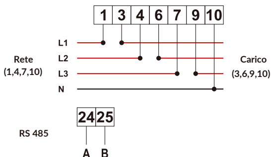
Figura 7.9 Contatore CHINT
