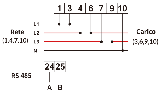
Figura 7.28 Contatore CHINT
