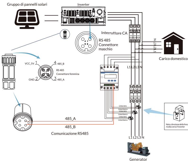
Figura 7.16 Schema di collegamento del contatore CHINT
