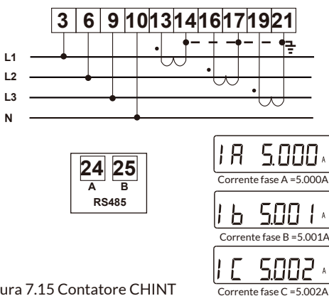
Figura 7.15 Contatore CHINT
